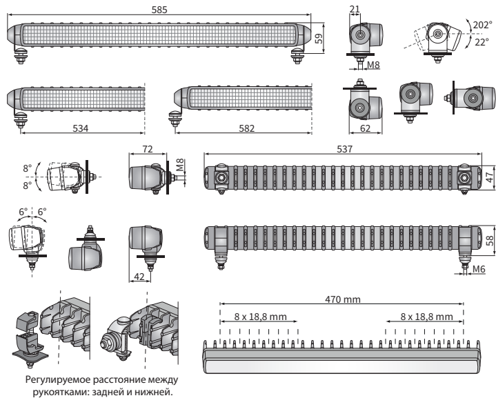
Освещенность в 1 люкс позволяет читать текст в газете Установка фары: 8° к вертикали выс.2,5м
